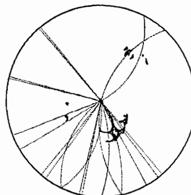
Interférences radar
